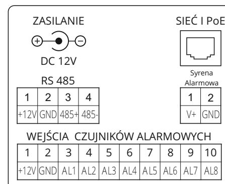
Montaż stacji GR-IS11-WA
