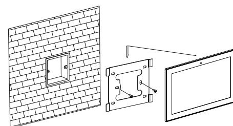
Montaż stacji GR-IS11-WA
