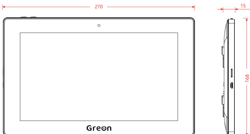
Wymiary panelu wewnętrznego GR-IS11-WA
